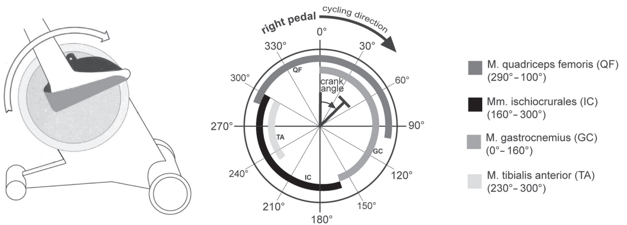
Abb. 1: Stimulationswinkel FES-LCE. Während der Rotationsbewegung am Bewegungstrainer werden die einzelnen Muskeln in den jeweiligen Winkelgraden stimuliert. Für das linke Pedal gelten die Winkelgrade wie abgebildet um 180° rotiert.
